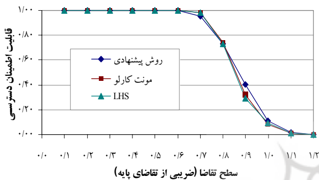
شکل 3. مقایسه قابلیت اطمینان دسترسی زوج مبدأ - مقصد (1 و 4) از روش‌های مختلف
