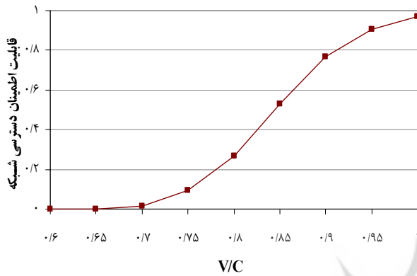
شکل ۷. نحوه تغییرات قابلیت اطمینان دسترسی شبکه برای مقادیر مختلف v_c
