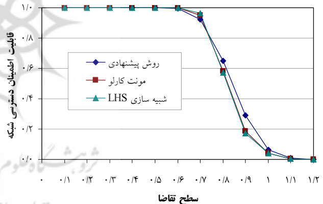
شکل 6. قابلیت اطمینان دسترسی شبکه از سه روش مختلف
