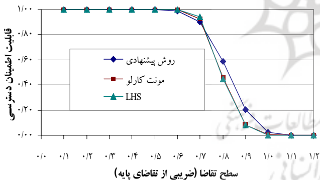
شکل 4. مقایسه قابلیت اطمینان دسترسی زوج مبدأ - مقصد (1 و 5) از روش‌های مختلف
