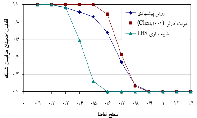
شکل 5. قابلیت اطمینان ظرفیت شبکه از سه روش مختلف
