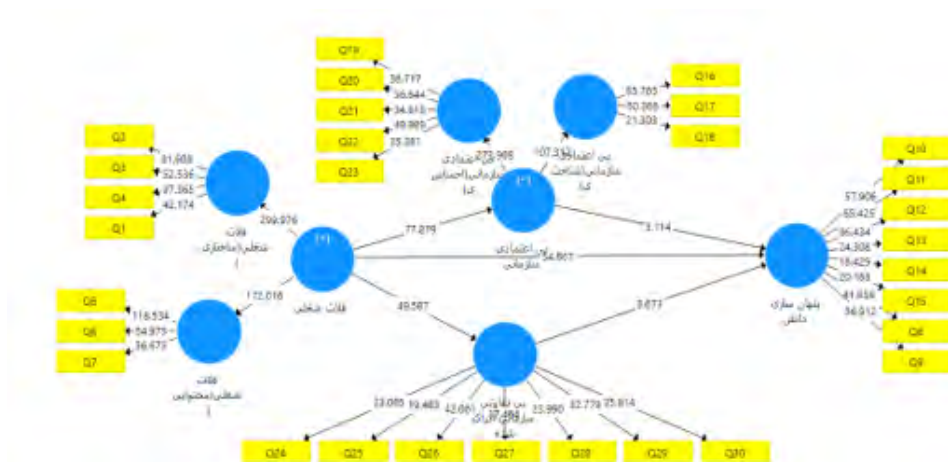
شکل ۴. مدل اجرا شده در نرم افزار pls به همراه آزمون آماری
