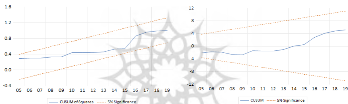
نمودار ۱. آزمون ثبات ضرایب CUSUM
