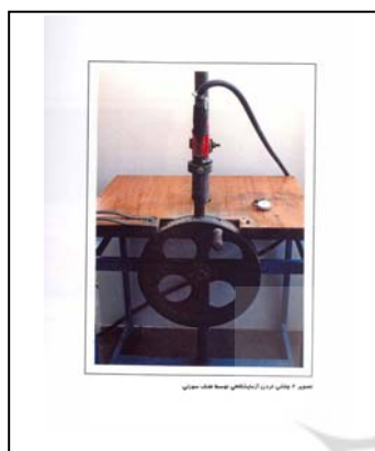
شکل 1. چکشی کردن آزمایشگاهی توسط تفنگ سوزنی
