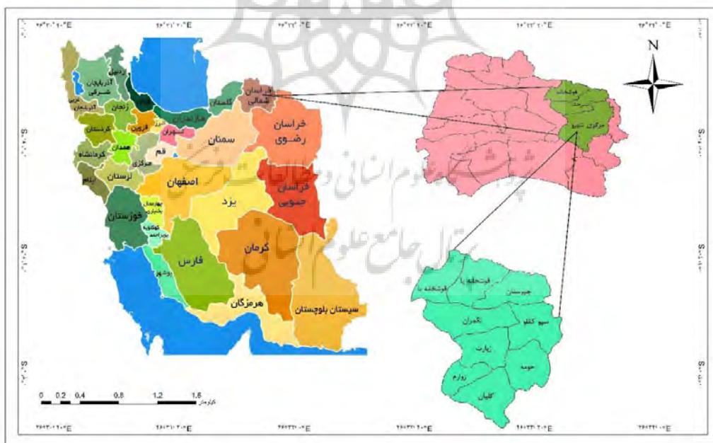
شکل ۲. موقعیت سیاسی شهرستان شیروان
