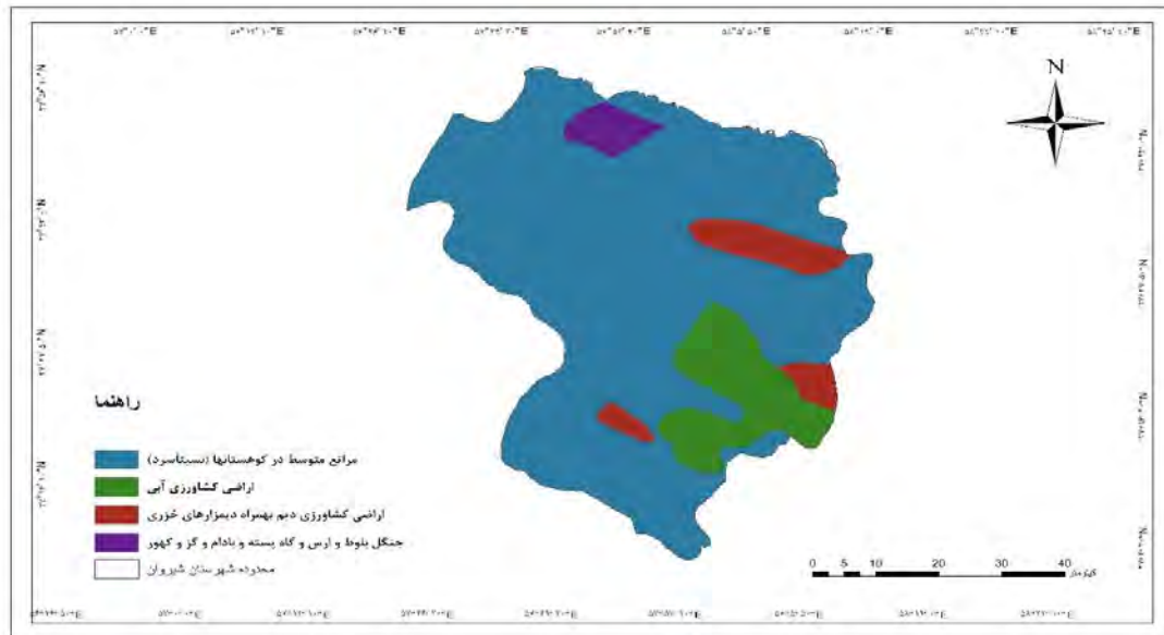
شکل ۳. پراکندگی پوشش گیاهی شهرستان شیروان
