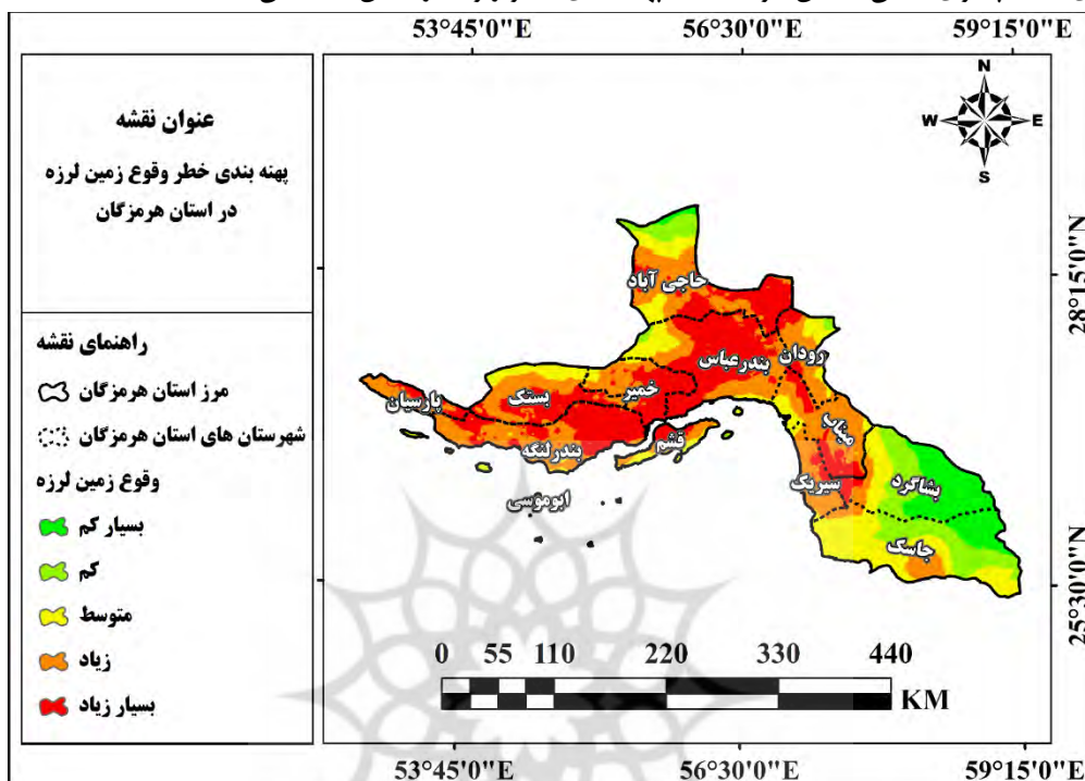
شکل ۱۹: نقشه پهنه‌بندی خطر وقوع زمین لرزه استان هرمزگان
