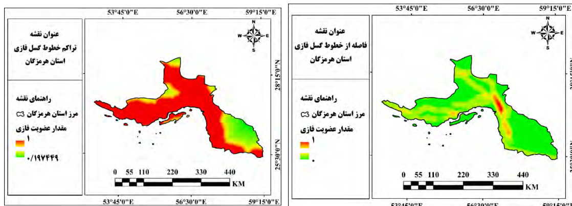
شکل ۸: نقشه فازی فاصله از خطوط گسل
