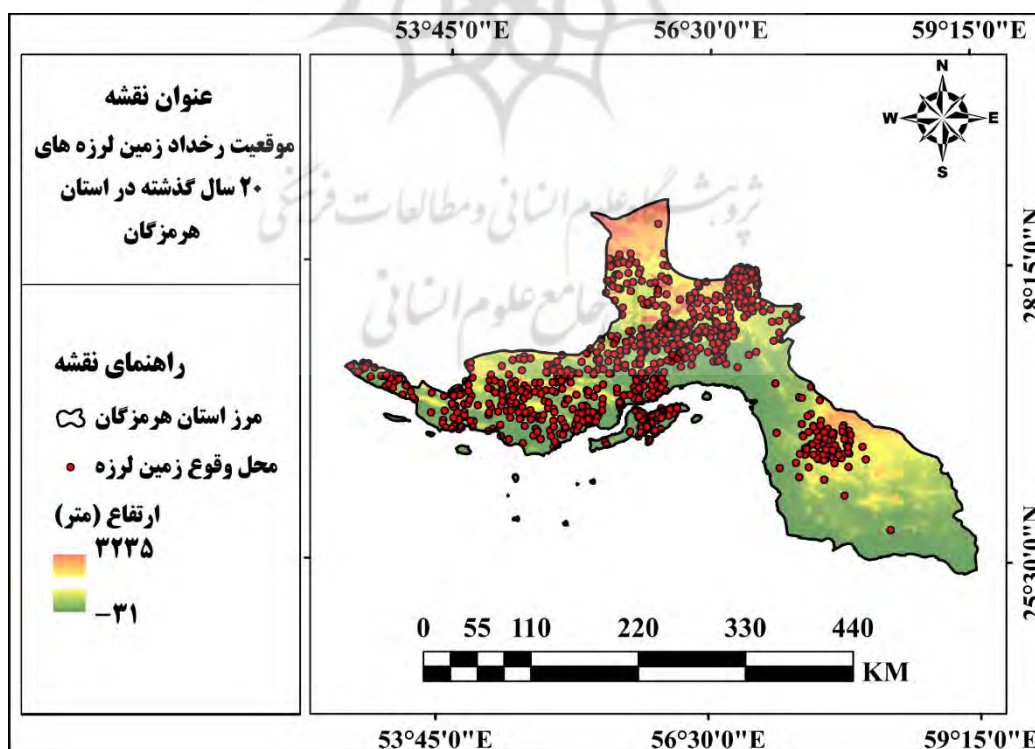
شکل ۱۰: نقشه پراکنش نقاط وقوع زمین لرزه در ۲۰ سال گذشته
