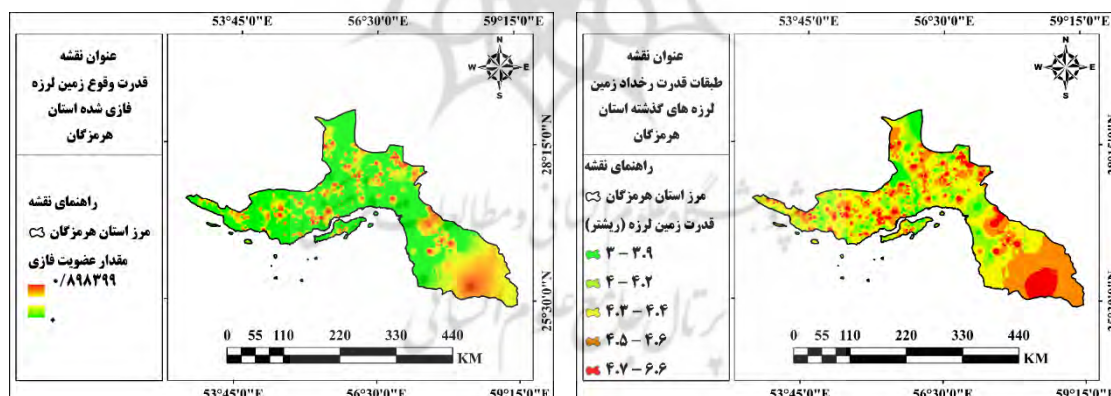
شکل ۱۴: نقشه فازی قدرت وقوع زمین‌لرزه‌های ۲۰ سال اخیر
