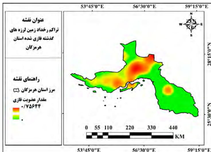
شکل ۱۸: نقشه فازی نقشه تراکم نقاط وقوع زمین‌لرزه‌های ۲۰ سال اخیر
