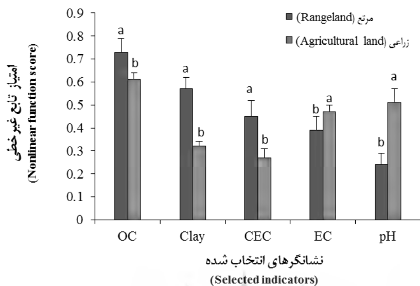
شکل ۳- مقادیر امتیازهای داده شده به نشانگرهای انتخاب شده برای MDS با استفاده از تابع غیر خطی
