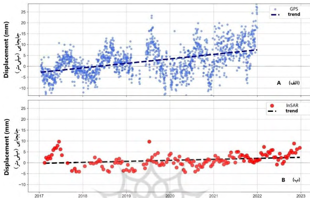
شکل ۴ - مقایسه جابجایی حاصل از GPS (الف) و InSAR (ب) در ایستگاه سرخس Fig. 4. Comparison of displacement obtained from GPS (a) and InSAR (b) at Sarakhs station
