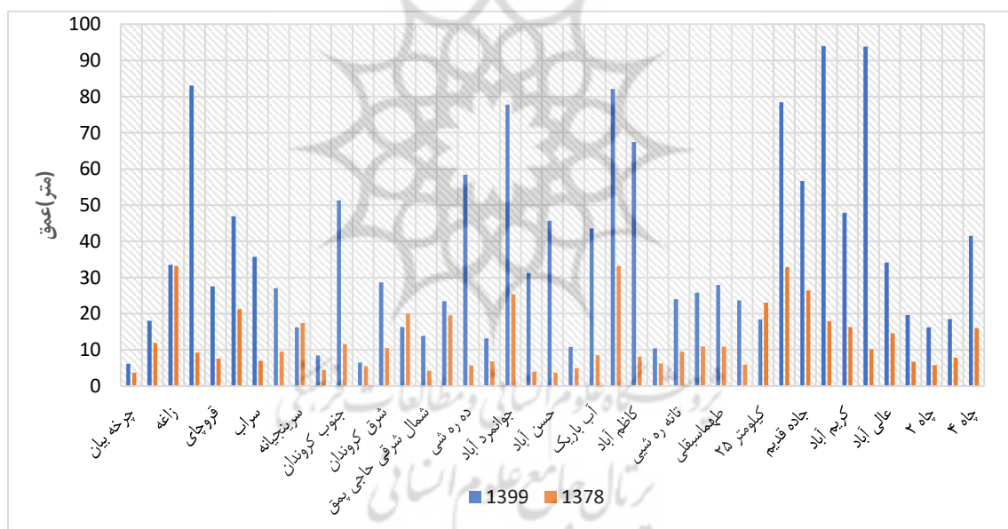
شکل ۸. نمودار سطح تراز آب زیرزمینی دشت دهگلان طی دو بازه زمانی ۲۰۰۰ و ۲۰۲۱
