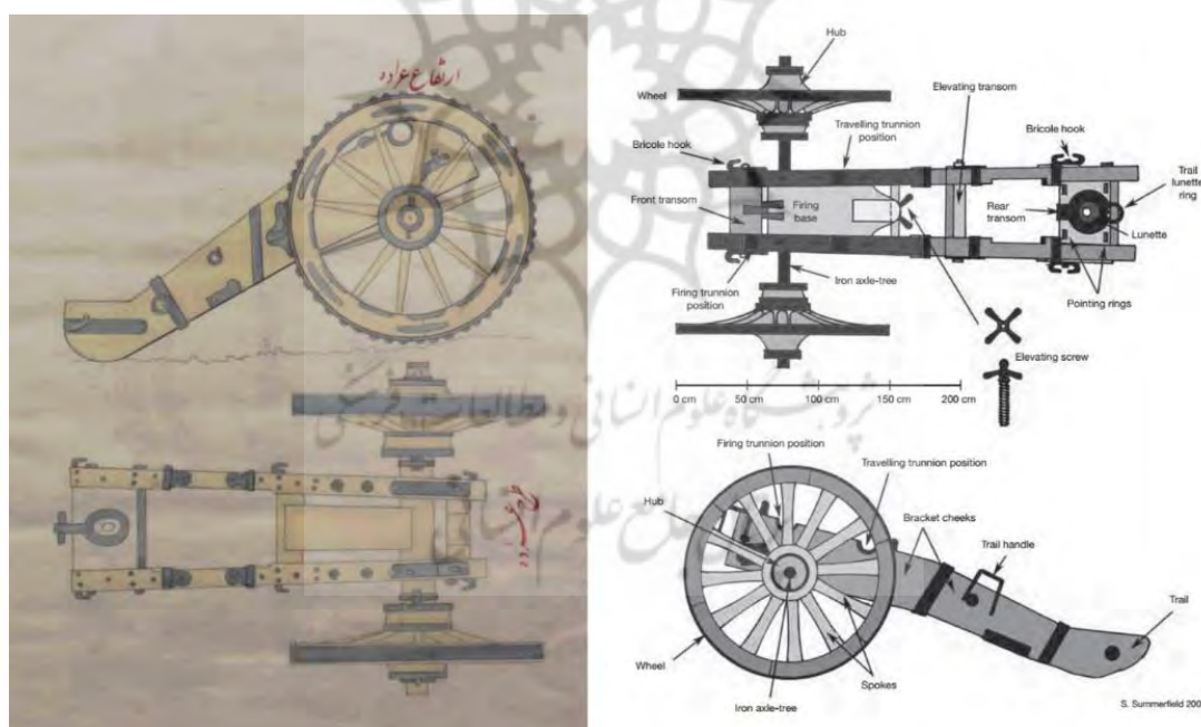
شکل ۳. چپ: عراده قیس (مهندس تبریزی، ۱۲۵۶: ۱۰۹)؛ راست: هویتزر فرانسوی گنپیروال مربوط به اوایل قرن نوزدهم میلادی. (Dawson & others, 2007: 21)
