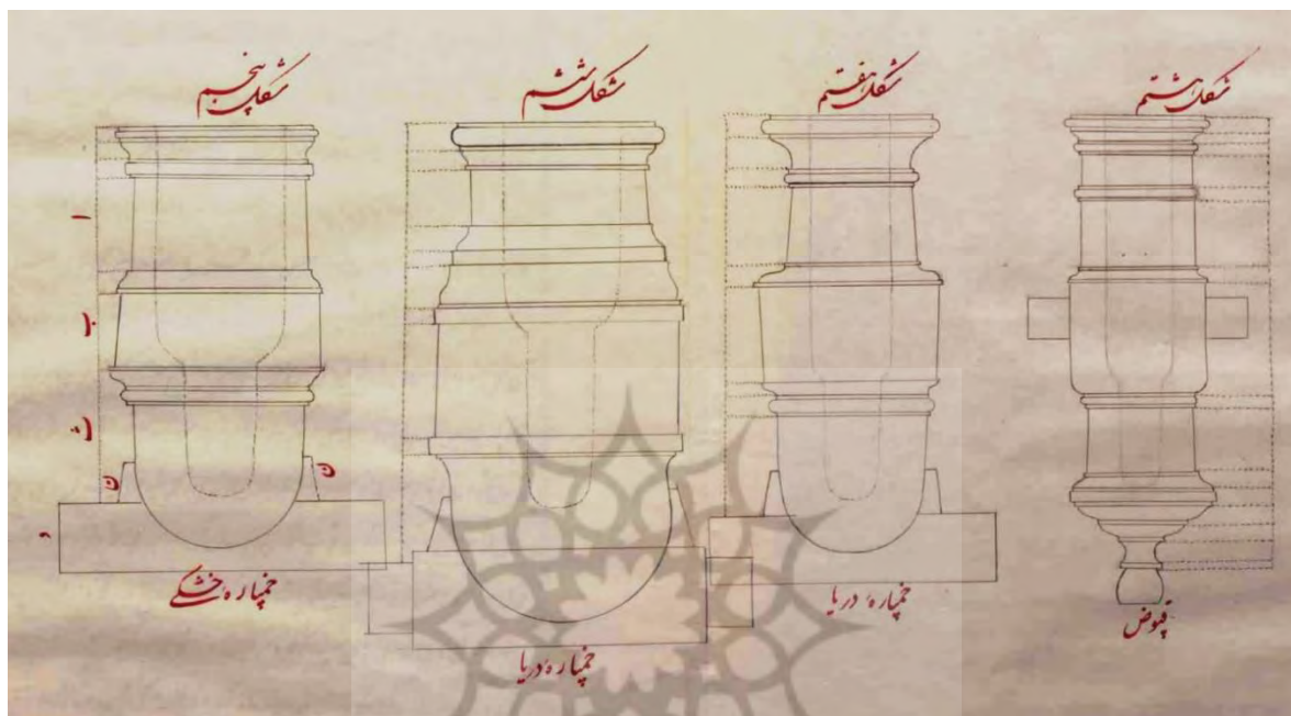
شکل ۱. از راست به چپ قپوض با بازوی میانی، دو خمپاره دریا و خمپاره خشکی با بازوهای تهتانی (مهندس تبریزی، ۱۲۵۶: ۴۹)
