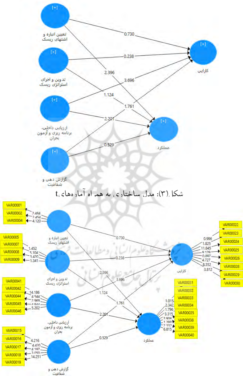
شکل (۴): نتایج آزمون t مدل اصلاح شده
