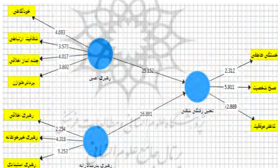
شکل ۴ - مدل ترسیم شده همراه با مقادیر آماره T برای فرضیه‌های تحقیق
