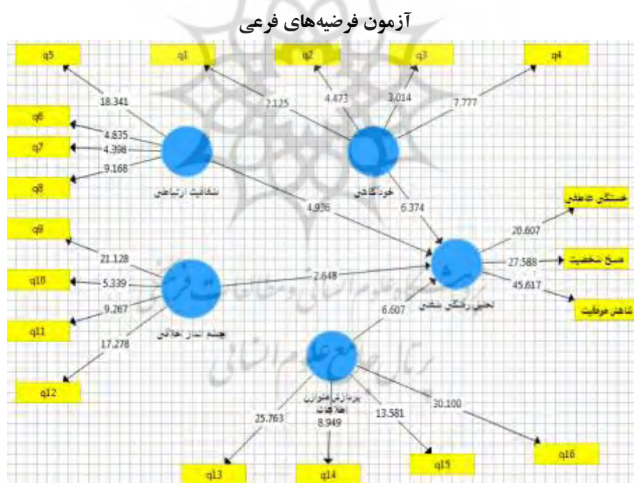
شکل ۷- مدل ترسیم شده همراه با مقادیر آماره T برای فرضیه‌های فرعی تحقیق
