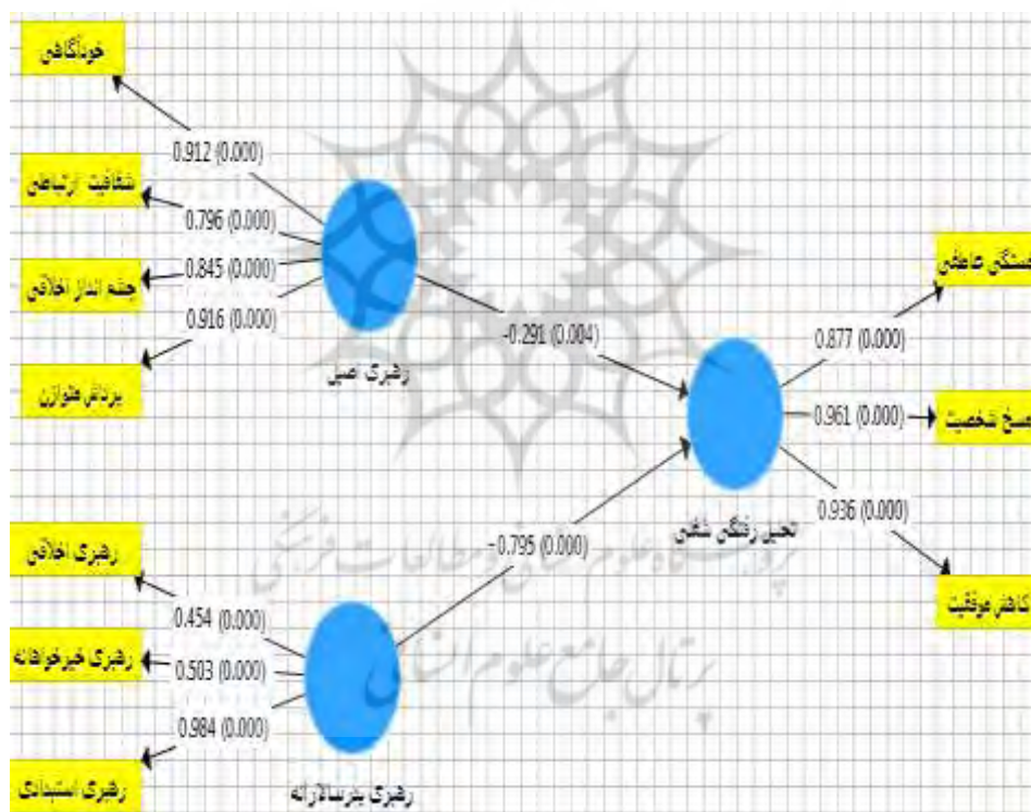
شکل ۵ - مدل ترسیم شده همراه با مقادیر P -value و ضرایب استاندارد فرضیه‌های تحقیق
