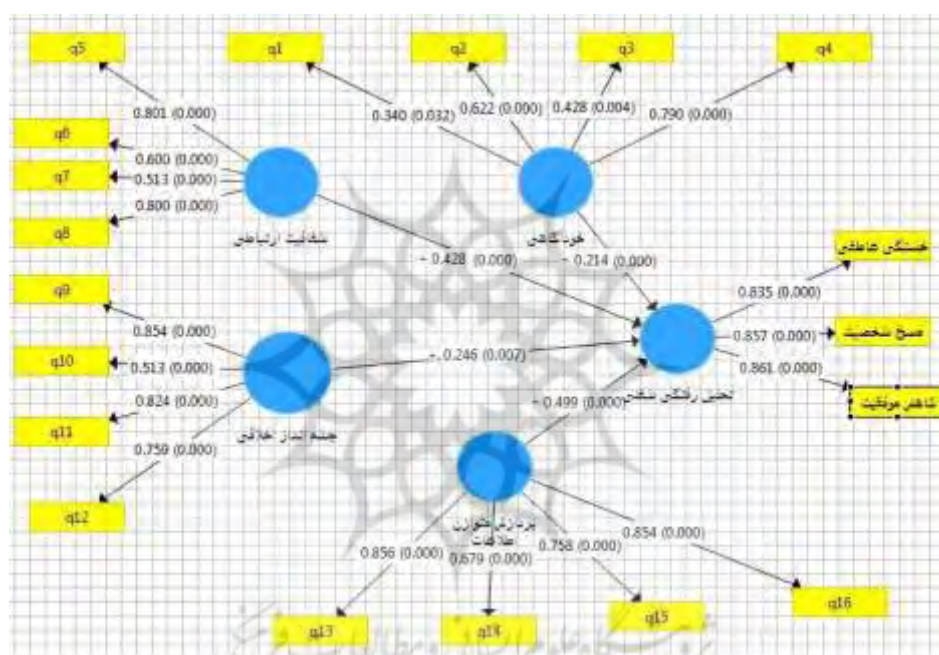
شکل ۸- مدل ترسیم شده همراه با مقادیر P-value و ضرایب استاندارد فرضیه‌های فرعی تحقیق
