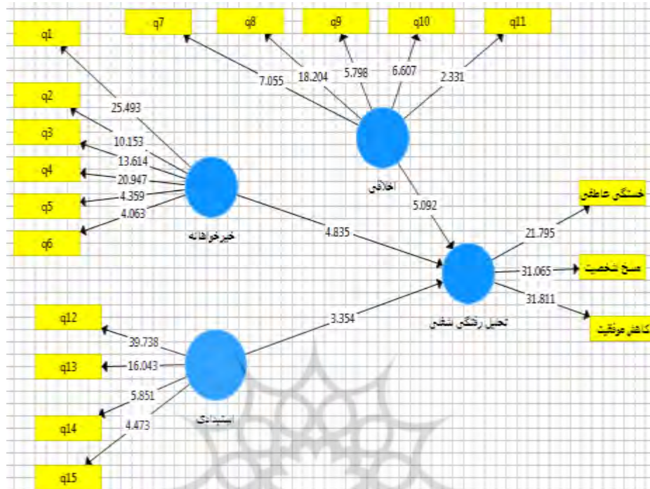
شکل ۹- مدل ترسیم شده همراه با مقادیر آماره T برای فرضیه‌های فرعی تحقیق
