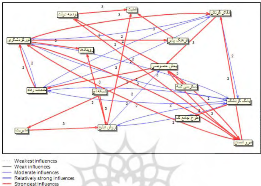
شکل ۴. گراف ماتریس تأثیر مستقیم
