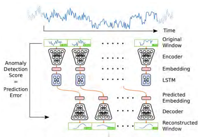
شکل ۳. مدل VAE-LSTM در توالی K پنجره زمانی
