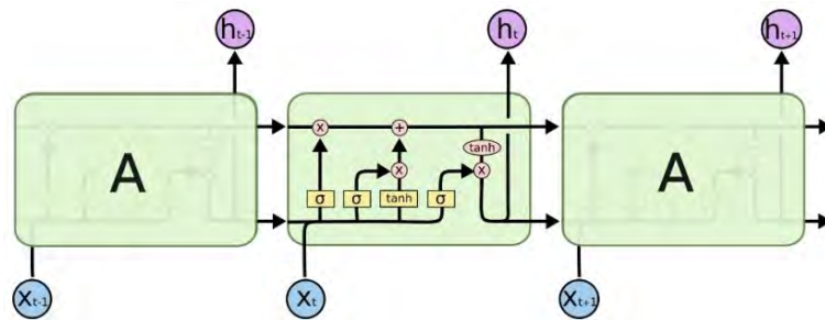
شکل ۱. ماژول تکرار شونده در مدل LSTM
