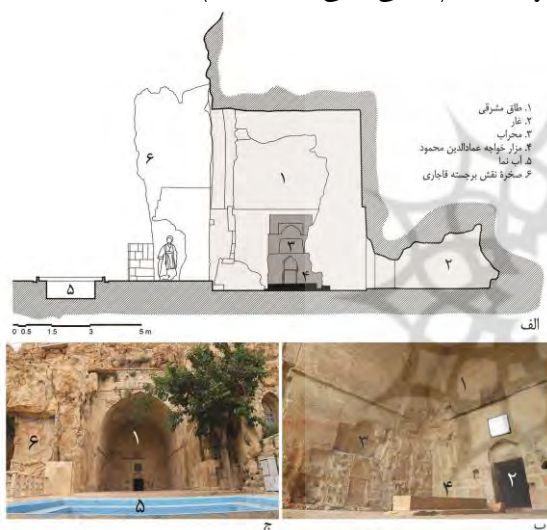
تصویر ۳- مقطع طاق مشرقی، سنگ مزار و محراب آن (نگارنده).
