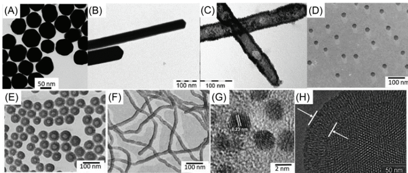
شکل ۵. تصاویر میکروسکوپ الکترونی عبوری از الف) نانوذرات طلا، ب) نانومیله‌های مسی، پ) مایسل‌های پسهاری، ت) وزیکول‌ها، ث) مایسل کرم مانند، ج) تصویر-میکروسکوپ الکترونی عبوری با قدرت تفکیک بالا از تیول پوشیده با نانوذرات طلا و چ) یک نانومواد مزوپور می‌شود (D.R. Baer, May 2010)
