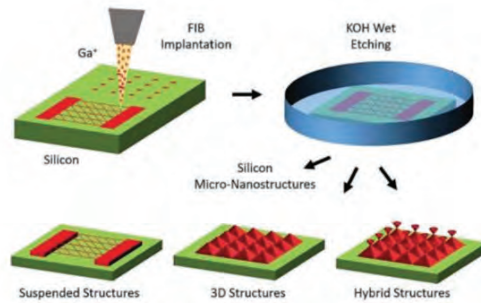
شکل ۲. نمودار شماتیک از ساخت ریز نانو ساختارهای سه بعدی با یک پرتو یونی از طریق ساختار Si. این شامل کاشت در Si از طریق لیتوگرافی Ga FIB و حکاکی ماسک با وضوح نانومتر، حکاکی مرطوب ناهمسانگرد بعدی در محلول KOH و ساخت ریز نانو ساختارهای Si از طریق حذف انتخابی ناحیه کاشته نشده است
