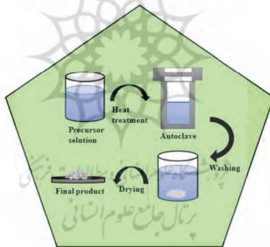
شکل ۴. نمودار شماتیک روش سنتز گرمایی (Abid et al., 2022)
