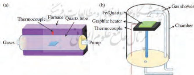
شکل ۳. تصویر شماتیک روش سنتز گرمایی (Abid et al., 2022)
