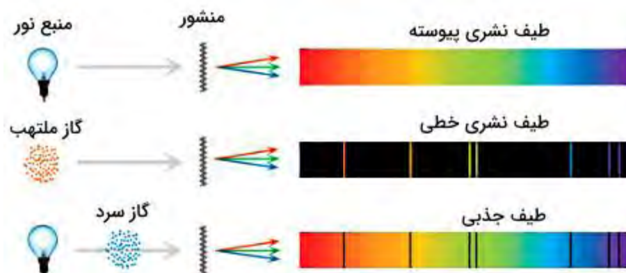
شکل ۲: نحوه تشکیل طیف نثری پیوسته، خطی و طیف جذبی (برگرفته از سایت فرادرس)
