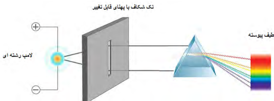
شکل ۵: طرح واره آزمایش تشکیل طیف پیوسته از یک لامپ رشته ای
