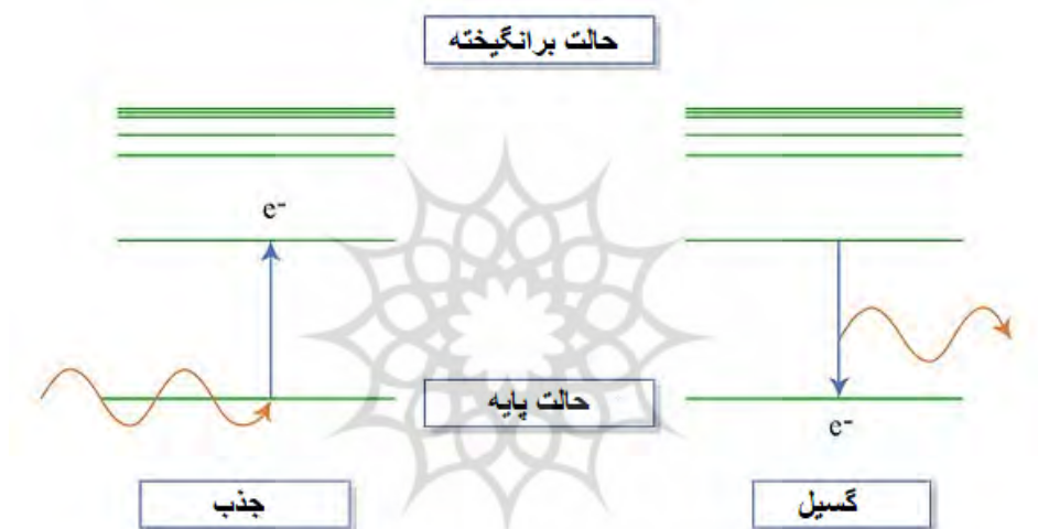
شکل ۳: جذب و گسیل اتمی در حالت پایه و برانگیخته
