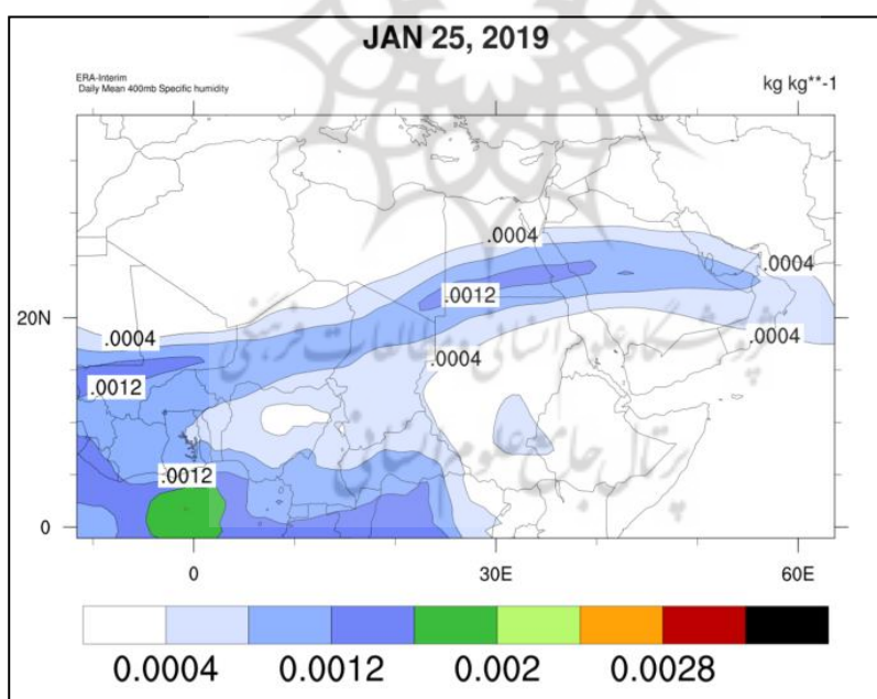
ب: رودخانه‌ای اتمسفری ۲۵ ژانویه ۲۰۱۹
