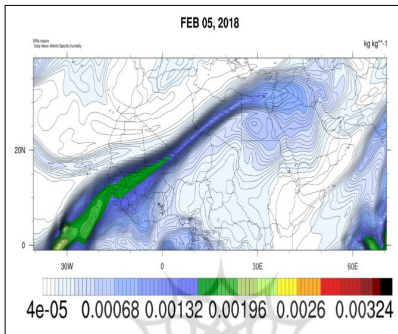
الف: رودخانه‌ای اتمسفری ۵ فوریه ۲۰۱۸
