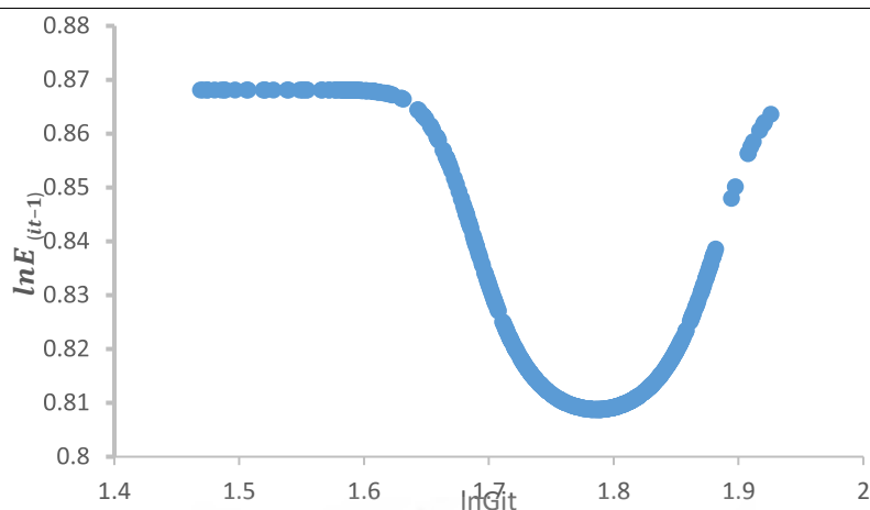
نمودار (۲): ضرایب همگرایی بتای شرطی
