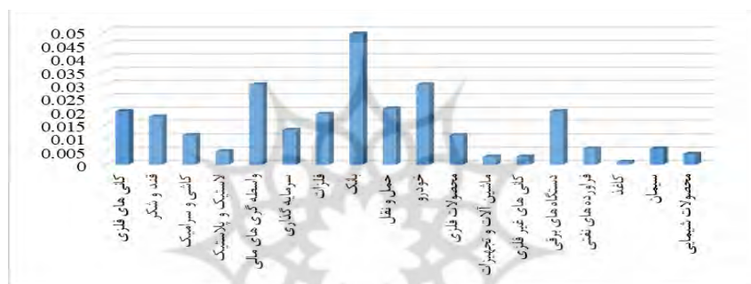
شکل ۳. مقایسه ضریب احساس گروه‌های بورسی بازار بورس اوراق بهادار تهران در مدل SDF رفتاری
