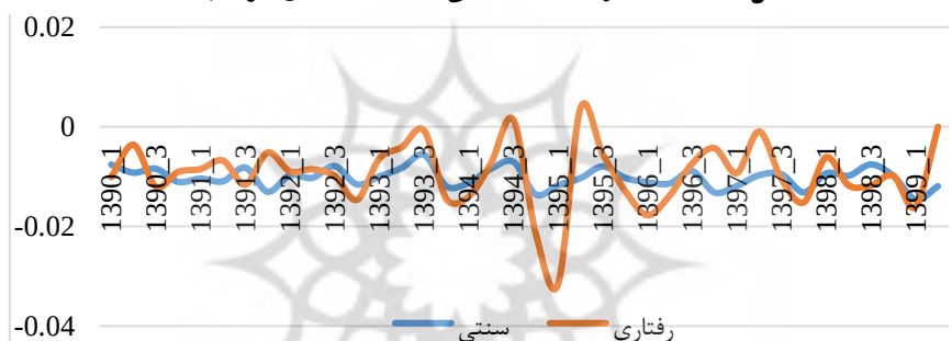
شکل ۵. مقایسه نمودار SDF سنتی و SDF رفتاری گروه بانک
