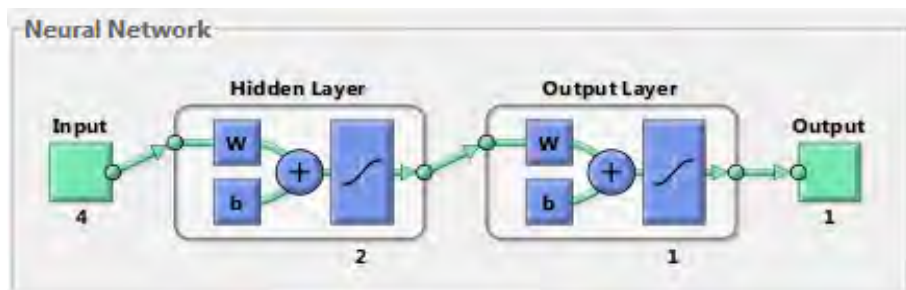
شکل ۲. ساختار شبکه عصبی مصنوعی با الگوریتم لونیگ - مارکووار به منظور پیش‌بینی مصرف گاز صنایع کشور
