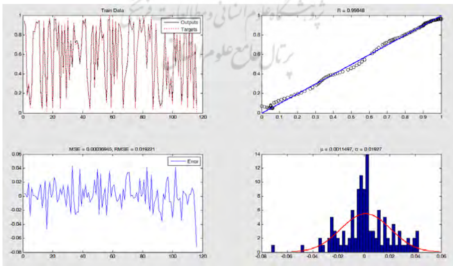
شکل ۹. نتایج اجرای شبکه عصبی مصنوعی ترکیب شده با الگوریتم ژنتیک در داده‌های آموزش برای ۱۵۰ تکرار
