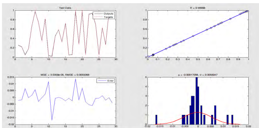
شکل ۵. نتایج به‌دست آمده برای داده‌های تست شبکه عصبی پرسپترون چندلایه با دو نورون
