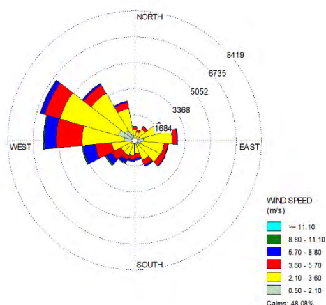
شکل ۲. گلبد مروداشت برای سال‌های ۲۰۱۲ تا ۲۰۲۱ Figure 2. Windrose of Marvdasht for 2012-2021
