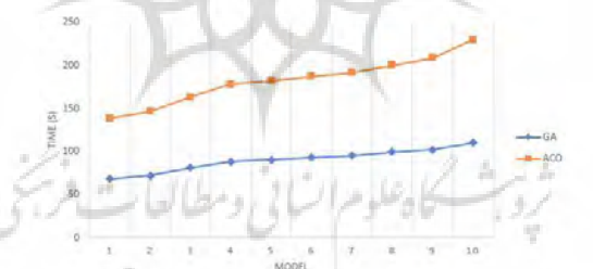
شکل ۷. مقایسه زمان اجرای کلی سیستم با استفاده از دو الگوریتم
