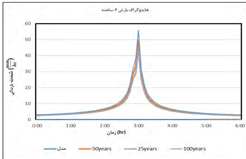
شکل (۱۳): هائیتوگراف بارش ۶ ساعته با دوره بازگشت‌های مختلف
