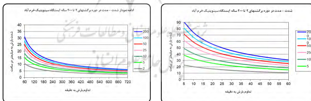
شکل (۱۲): نمودار شدت - مدت در دوره برگشتی ۲ تا ۲۰۰ ساله ایستگاه سینوپتیک خرم آباد
