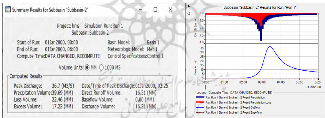
شکل (۱۴): خروجی شبیه سازی با دوره بازگشت ۲۵ سال
