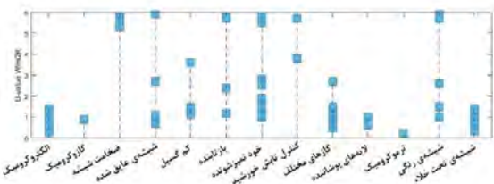
شکل ۱۰. مقایسه میانگین ضریب انتقال حرارت بر اساس گزارش‌های تجاری منتشر شده (IQ Glass, 2017 - NSG- Group, 2017)
