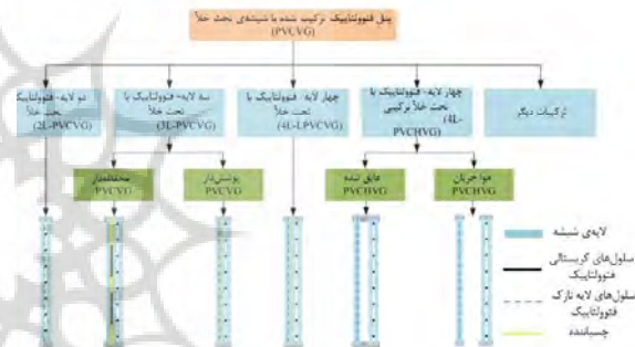
شکل ۹. طبقه‌بندی فتوولتائیک‌های ترکیب شده با شیشه‌ی تحت خلأ (Uddin et al., 2023)
