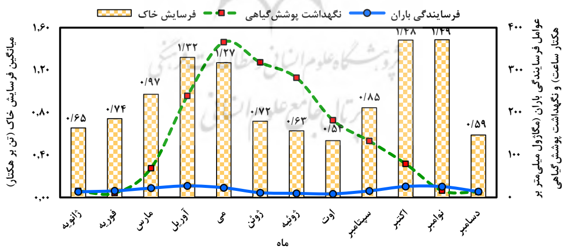
شکل ۷: ارتباط بین مقادیر میانگین فرسایش خاک، عوامل فرساینده گیاهی باران و نگهداشت پوشش گیاهی در مقیاس ماهانه بزرگ آبخیز دریای خزر
