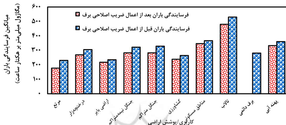
شکل ۴: تغییرات میانگین عامل فرساینده‌گی باران سالانه قبل و بعد از اعمال ضریب اصلاحی پوشش برف در کاربری‌ها/پوشش‌های مختلف اراضی بزرگ آبخیز دریای خزر
