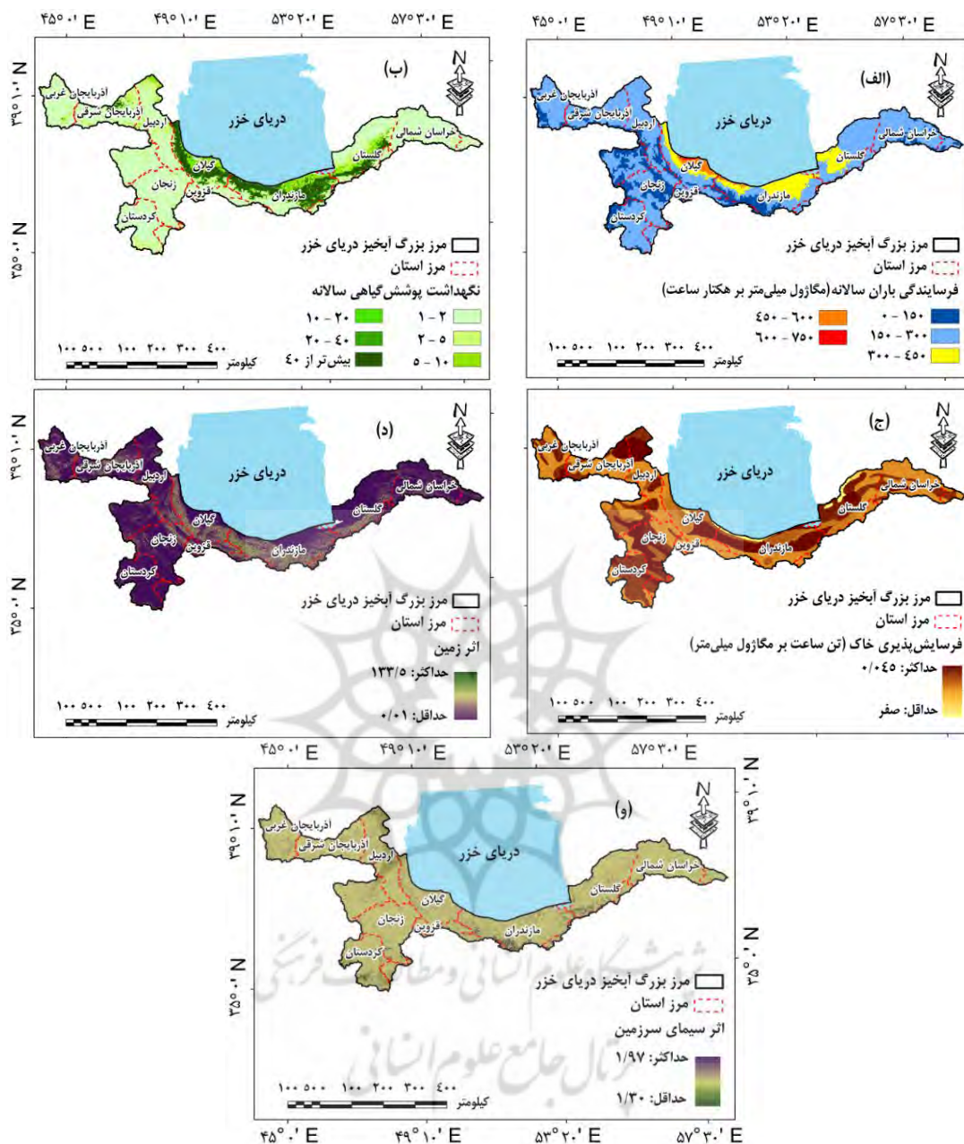
شکل ۵: نقشه‌های عوامل ورودی مدل G2 در بزرگ آبخیز دریای خزر (الف: عامل فرسایش پذیری باران (R); ب: عامل نگهداشت پوشش گیاهی (V); ج: عامل فرسایش پذیری خاک (S); د: عامل اثر زمین (T); و: عامل اثر سیمای سرزمین (L))
