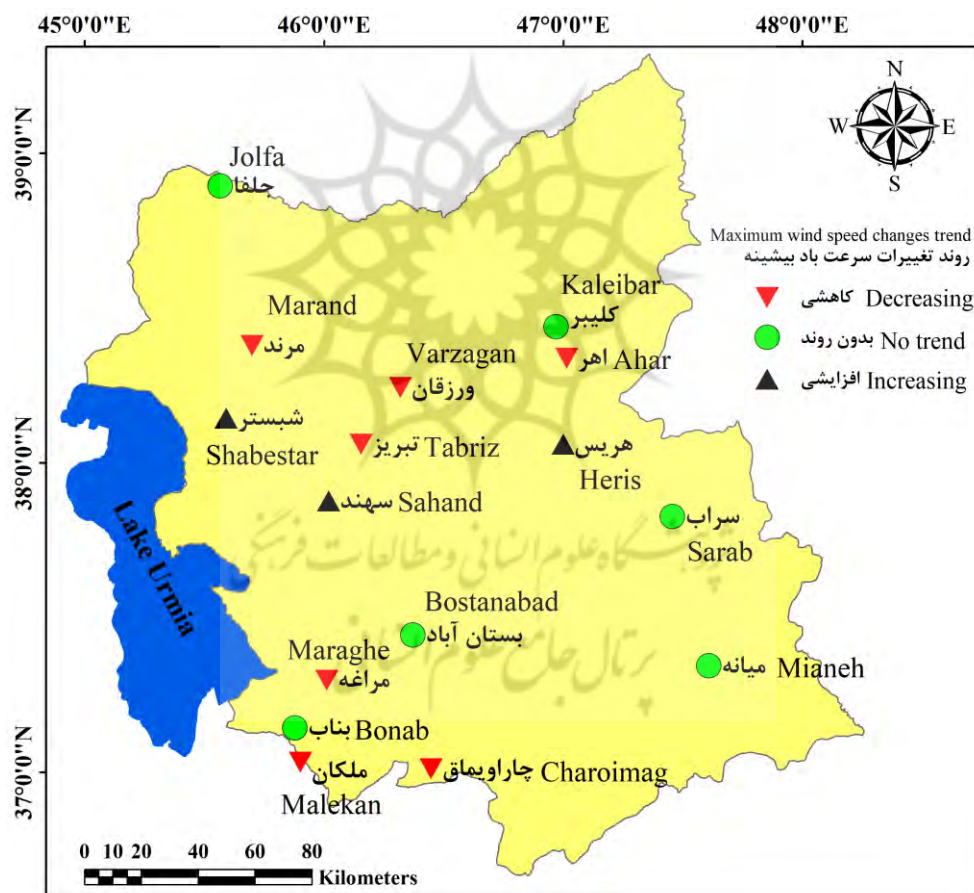
شکل ۳- روند تغییرات سرعت باد بیشینه در ایستگاه‌های همدیدی شرق دریاچه ارومیه
