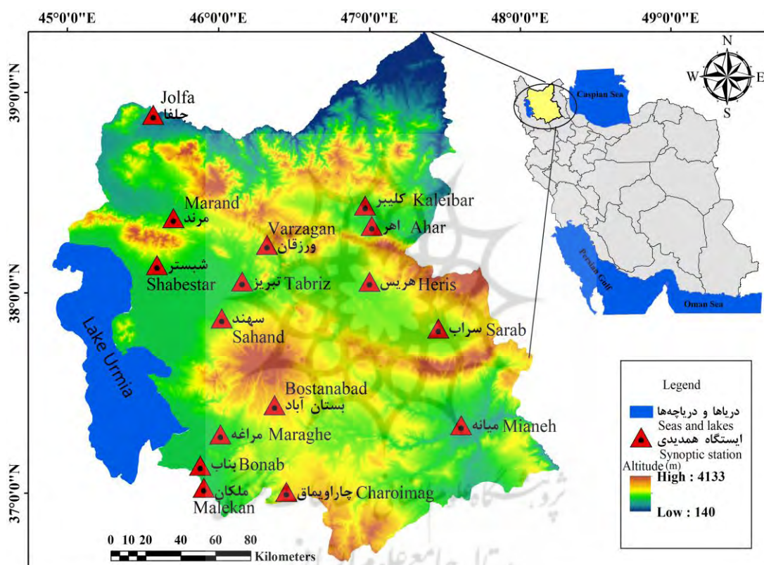
شکل ۱- موقعیت جغرافیایی ایستگاه‌های همیدی استان آذربایجان شرقی
