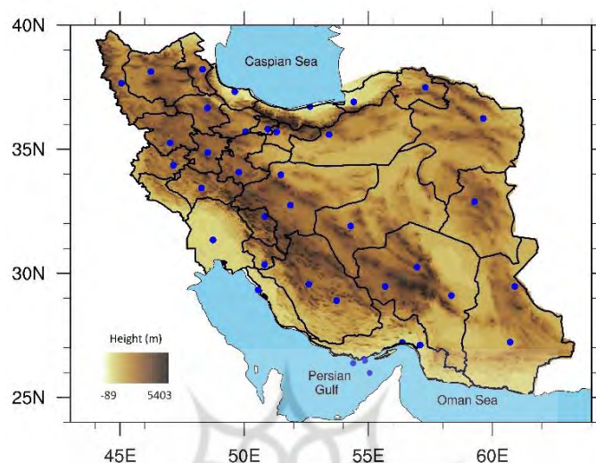
شکل ۱- موقعیت ایستگاه‌های همدیدی مورد مطالعه به همراه کوهساری منطقه
