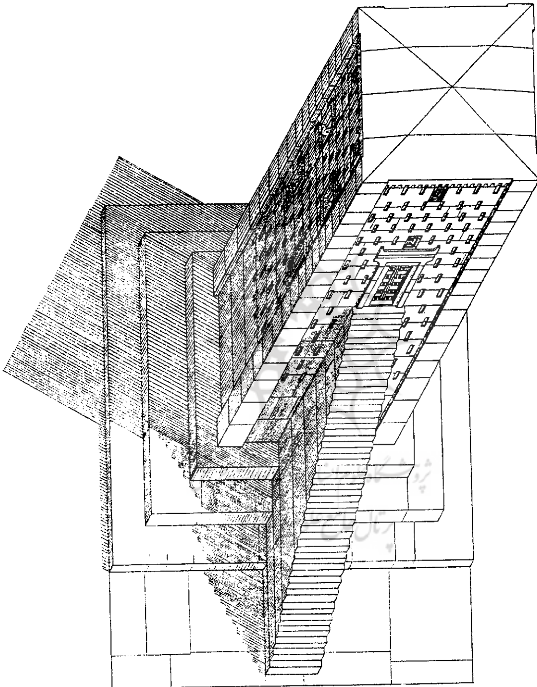
تصویر ۹- طرح بازسازی شده برج سنگی و پلکان آن
