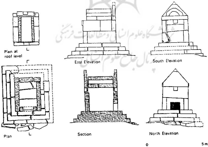
تصویر ۱۱- طرح بازسازی شده آرامگاه کوروش
