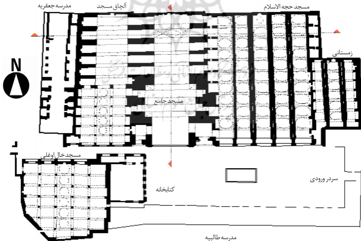
تصویر ۴. پلان وضع موجود مجموعه مسجد جامع کبیر تبریز. مأخذ: (آرشیو سازمان میراث فرهنگی، صنایع دستی و گردشگری استان آذربایجان شرقی)
