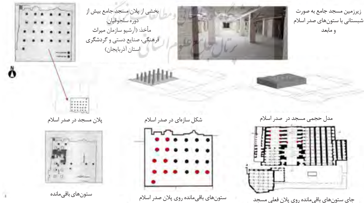
تصویر ۸. تصاویر، پلان‌ها و مدل حجمی مربوط به صدر اسلام.
