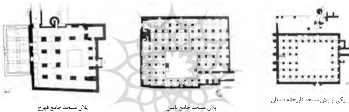
تصویر ۷. پلان سه مسجد دامغان، نایین، فهرج مربوط به صدر اسلام.
