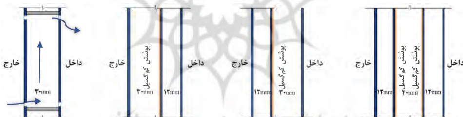
تصویر ۵: حالت شماره ۱: نمای تنفسی دولایه بدون پنجره دوجداره / حالات ۲، ۳، ۴: قرارگیری پنجره دوجداره در نمای تنفسی (عرض و ارتفاع بازشوها: ۶۰ سانتی‌متر).
