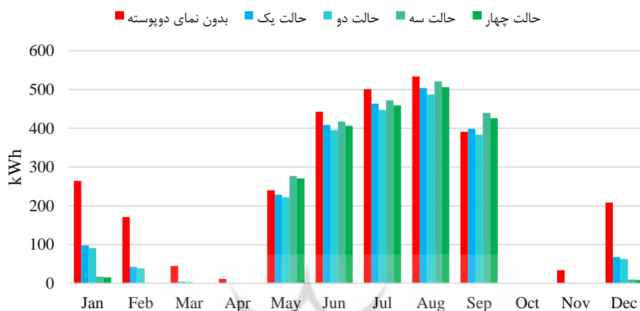
تصویر ۷: مجموع بار سرمایش و گرمایش حالت‌های مختلف
