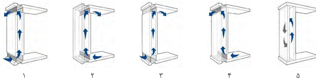
تصویر ۲: پنج حالت تهویه در نماهای دوپوسته مأخذ: (Jankovic & Goia, 2021)
