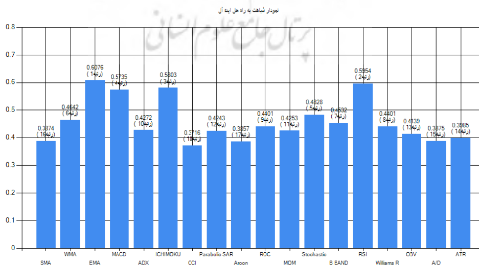
شکل ۱. نمودار شباهت به راه حل ایده‌آل شاخص‌های تکنیکال بر اساس نظرهای خبرگان
