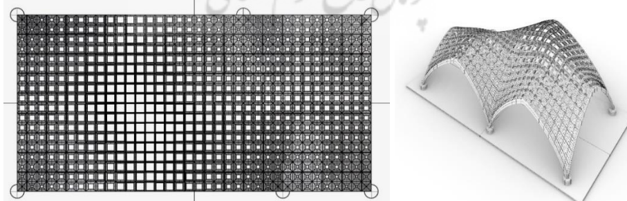
شکل ۱. آلاچیق با فرم قوسی شکل آزاد و طرح مشبک با اندازه‌های متنوع آن در پلان، خروجی از نرم‌افزار Rhinoceros.7.34. (پژوهشگران)
