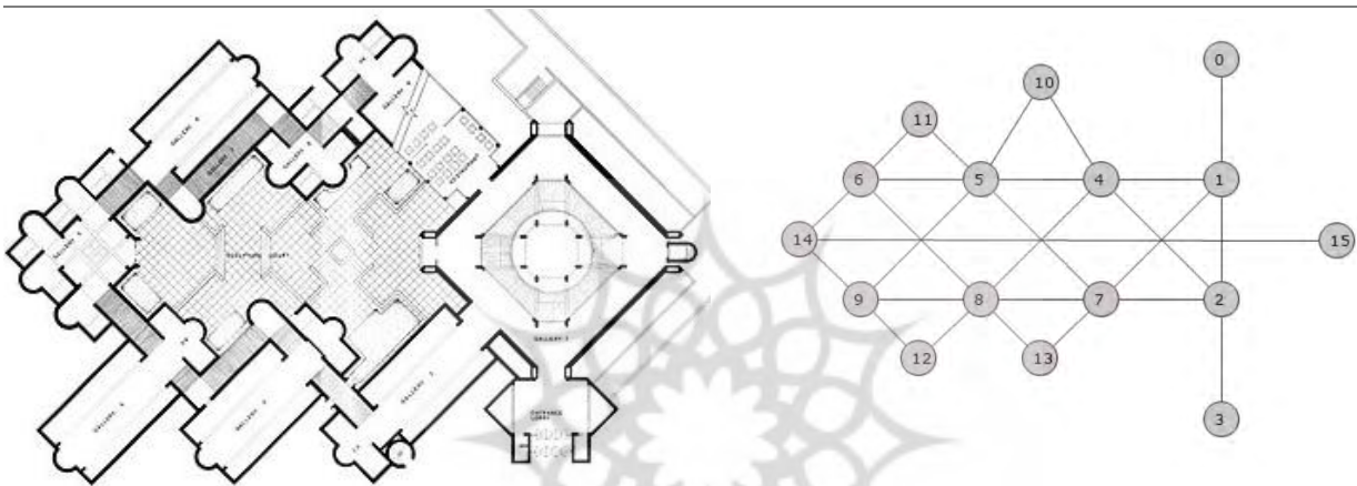
پلان و گراف موزه هنرهای معاصر تهران
