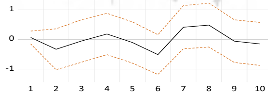
نمودار ۱۳- شوک شاخص اعتماد یکساله - بلندمدت
