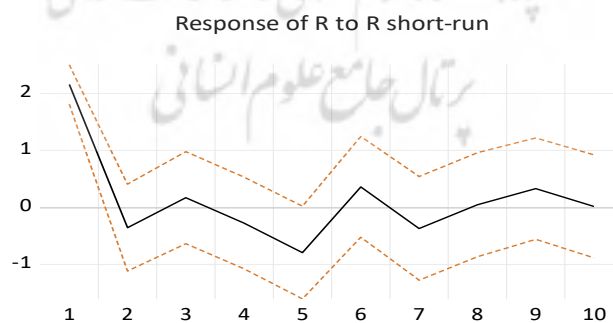
پژوهشگاه علوم انسانی و مطالعات فرهنگی Response of R to R short-run \pm 2 S.E.
