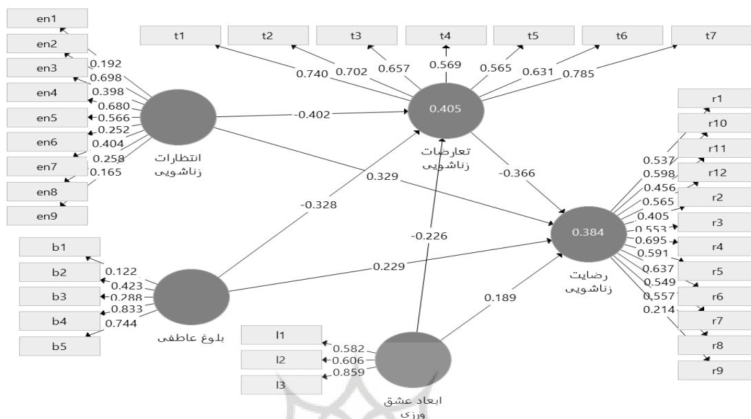
شکل ۱. ضرایب استاندارد شده مسیرهای مدل مفهومی پژوهش
