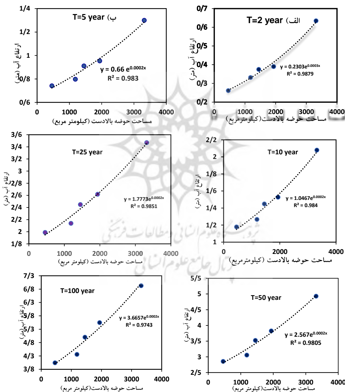
شکل ۴) ارتباط مساحت بالادست هر نقطه انتخابی با ارتفاع آب در ارتباط با دوره بازگشت‌های مختلف (۲، ۵، ۱۰، ۲۵، ۵۰، ۱۰۰ سال)
