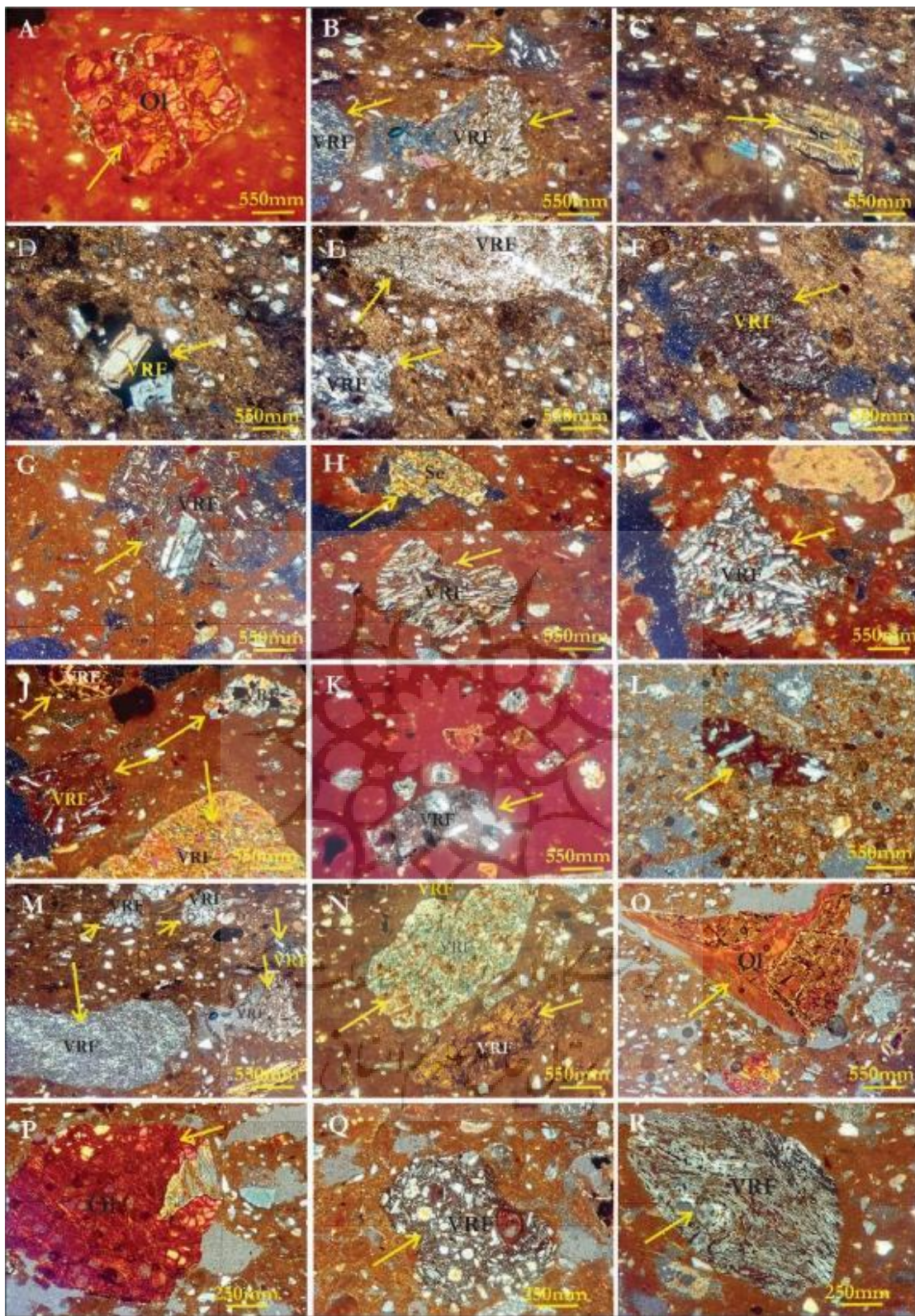
شکل ۶: تصاویر میکروسکوپی (نور پلاریزه متقاطع) از انواع خرده سنگ‌های آذرین (حد واسط و ولکانیکی) (VRF) و قطعات سنگی سربانتینت (Se) و کانی الیوین (OI) در بزرگنمایی‌های ۵X و ۱۰X.
