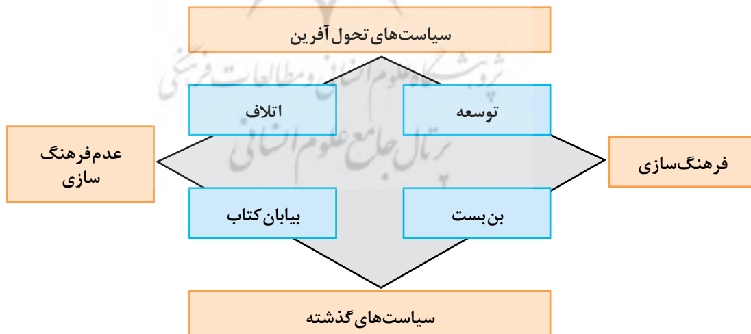
شکل ۱. ماتریس سناریو
