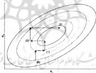
شکل ۱. نمونه‌ای از الگوریتم نمونه‌گیری گیبس به شکل دو بعدی از نقطه اولیه شروع و پس از سه تکرار تکمیل می‌شود.
