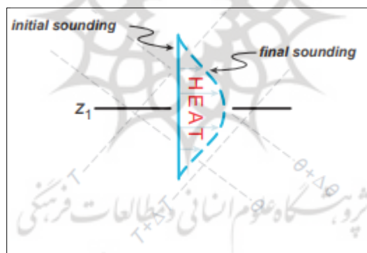
شکل (۸). نمودار ترمودینامیکی اثر گرمایش بی‌دررو دیفرانسیل در بررسی آهنگ کاهش دما را نشان می‌دهد
