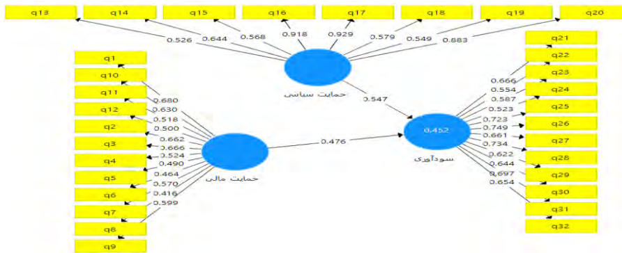
شکل (۱): مدل در حالت تخمین ضرایب استاندارد
