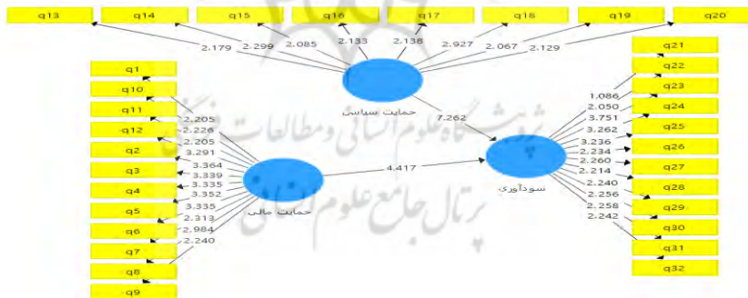
شکل (۲): مدل در حالت تخمین ضرایب معنی‌داری
