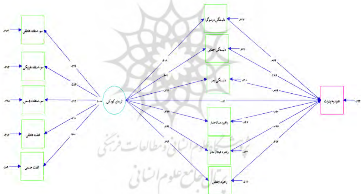
شکل ۲) تحلیل مدل ساختاری پژوهش با استفاده از روش بیشینه درست‌نمایی (ضرایب استاندارد)
