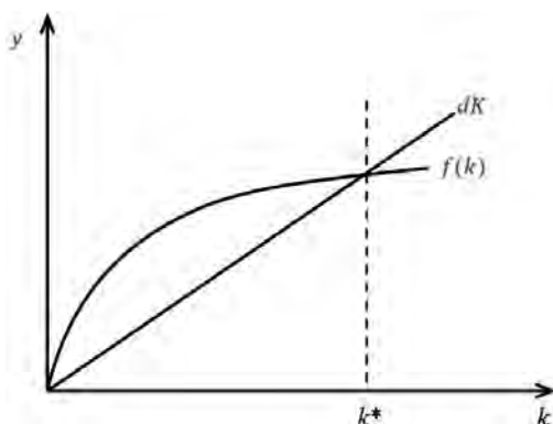
نمودار ۲. تابع تولید در مدل سولو به همراه تابع استهلاک (Solow, 1956: 70)
