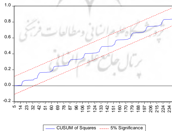
نمودار 2. آزمون CUSUMSQ
