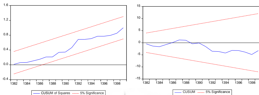
نمودار ۴. آزمون CUSUM و CUSUMQ در برآورد الگوی پژوهش در قالب نامتقارن منبع: یافته‌های پژوهش
