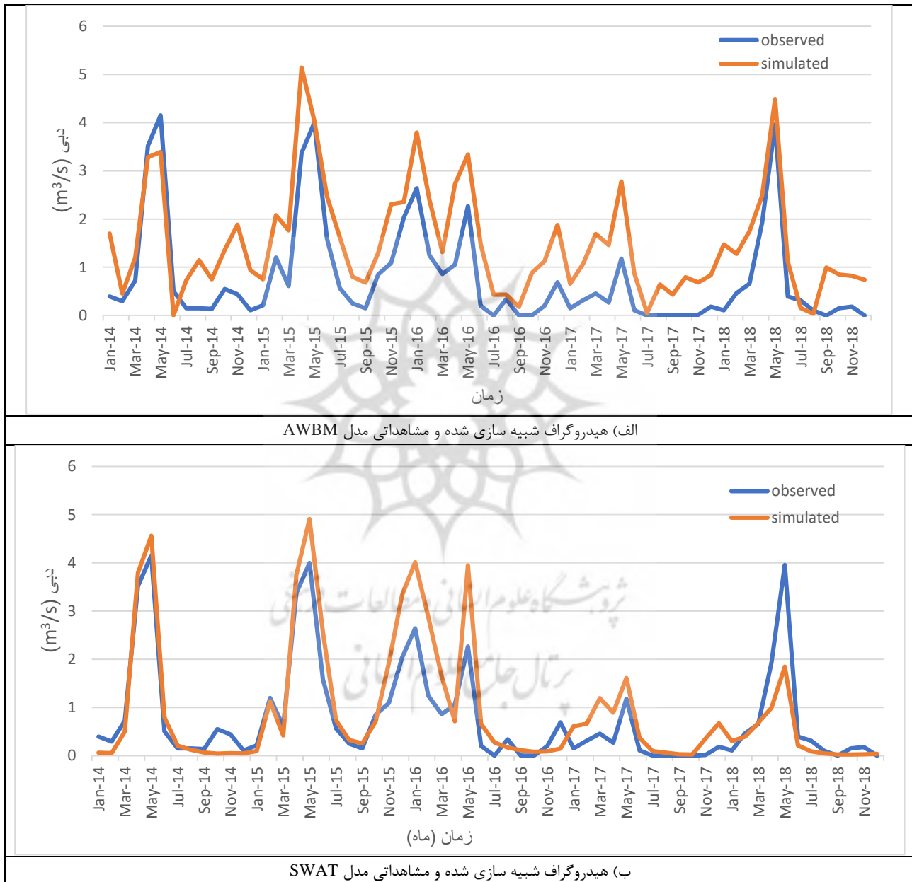
شکل ۵: هیدروگراف‌های شبیه‌سازی شده و مشاهداتی - رواناب ماهیانه در حوضه گمناب چای در دوره صحت‌سنجی مدل‌های مورد مطالعه
