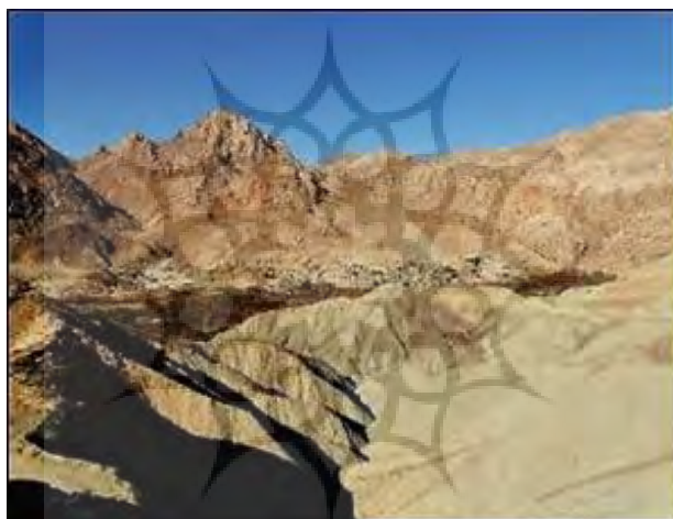
شکل ۱۲. بدلندهای روستای سرند در مارن‌های سازند بغمشاه
