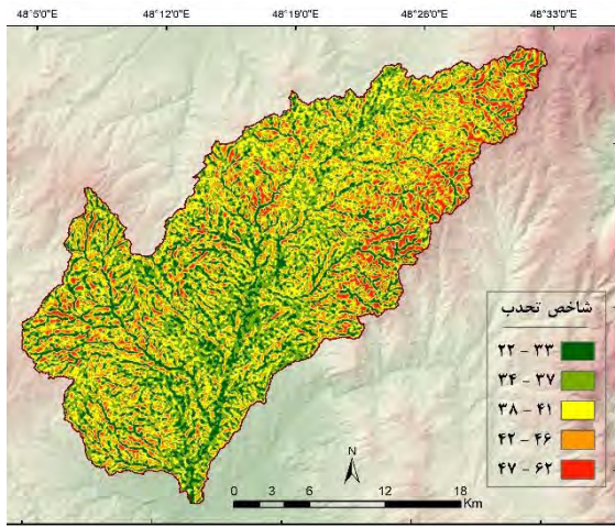
شکل ۵- تحدب سطح زمین در حوضه فیروزآباد
