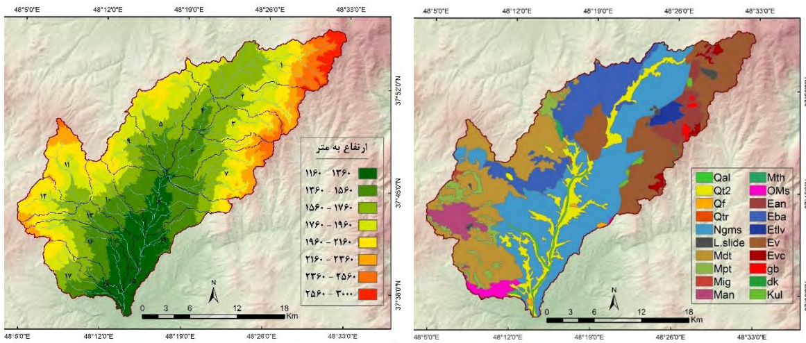
شکل ۱۴- سازندهای زمین‌شناسی در حوضه فیروزآباد
