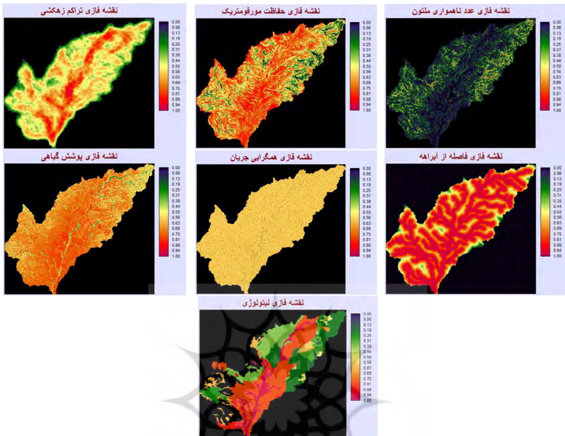
شکل ۱۶- نقشه‌های لایه‌های موضوعی مورد استفاده در پهنه‌بندی فرسایش حوضه فیروزآباد
