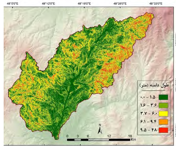
شکل ۴- توزیع طول دامنه در حوضه فیروزآباد
