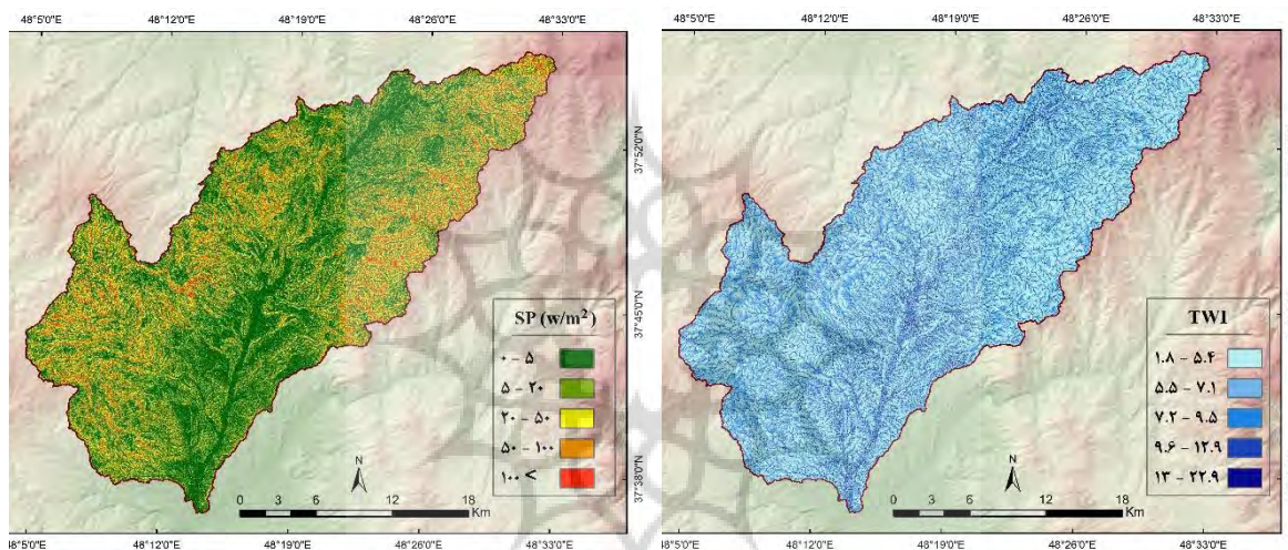
شکل ۷- شاخص توان رودخانه در حوضه فیروزآباد
