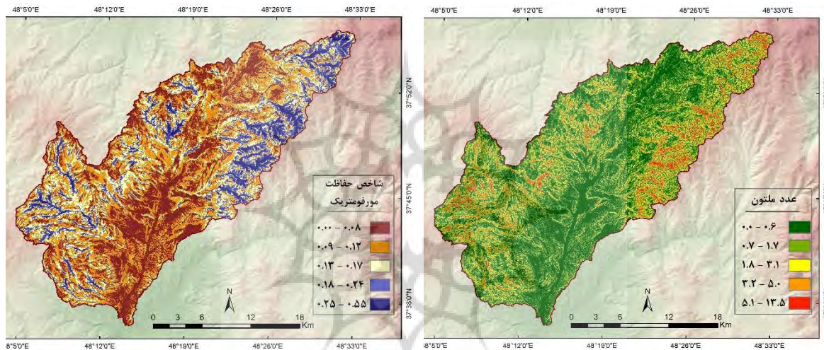
شکل ۹- شاخص حفاظت مورفومتریک در حوضه
