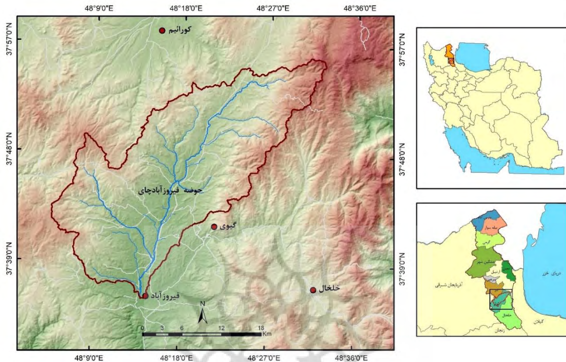
شکل ۱- موقعیت حوزه آبریز فیروزآبادچای در شمال غرب کشور
