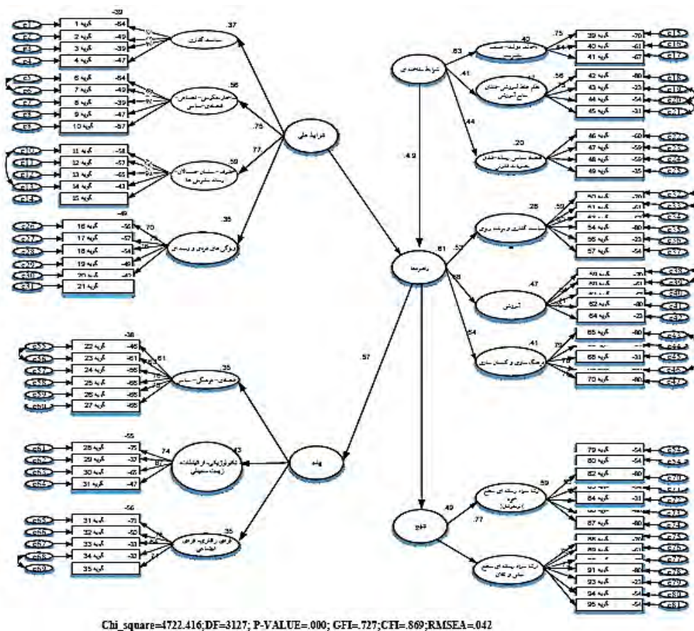
جدول ۴. تحلیل مسیر مدل پارادایمی پژوهش
